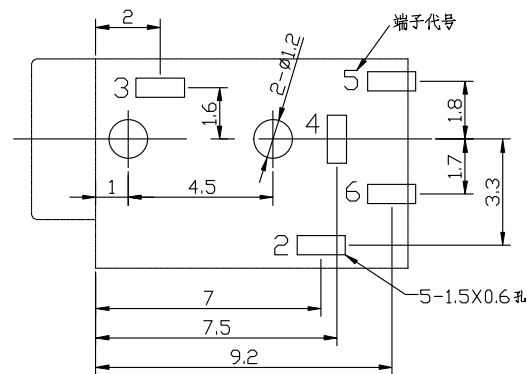
PCB, 开孔尺寸图 Top View
