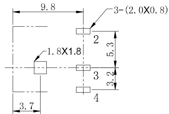
线路板开孔尺寸 P.C.B LAYOUT
