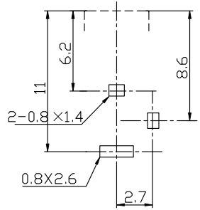
线路板开孔尺寸
